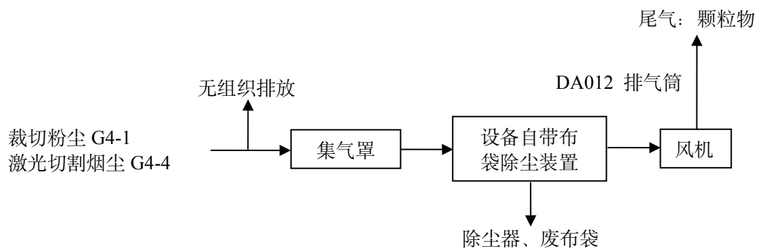
图 4-8 DA012 排气筒废气处理装置示意图
