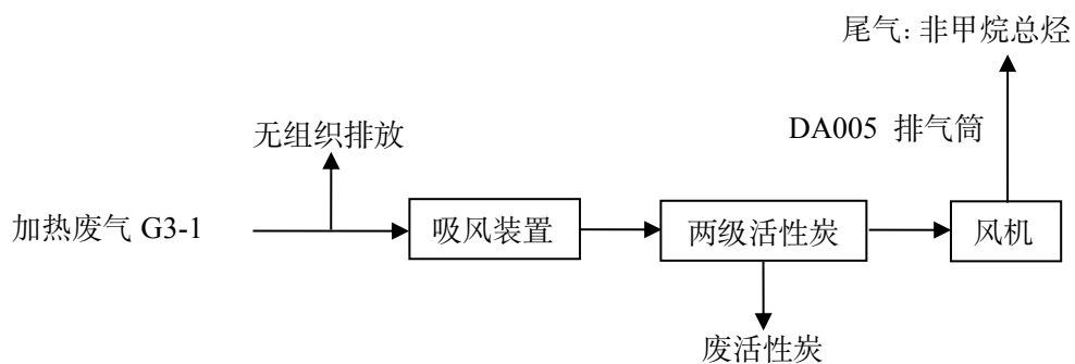
图 4-3 DA007 排气筒废气处理装置示意图
