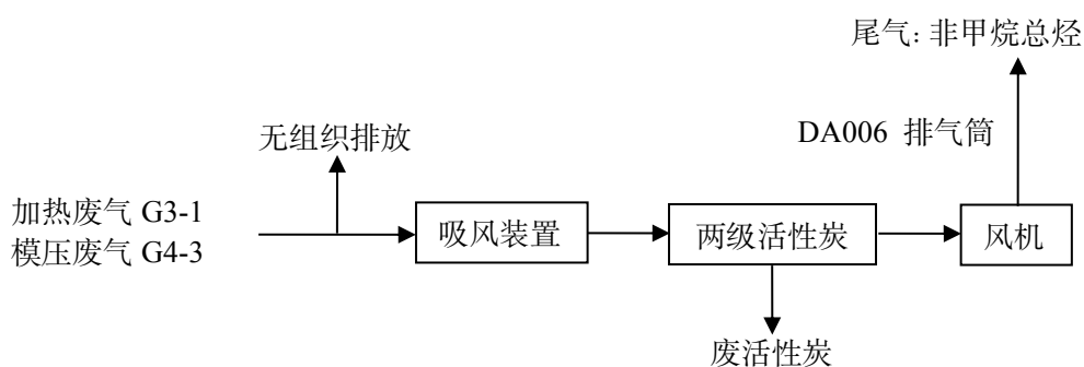
图 4-4 DA008 排气筒废气处理装置示意图
