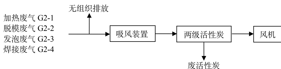
图 4-6 DA011 排气筒废气处理装置示意图
