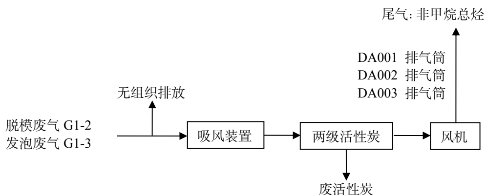
图 4-2 DA001、DA002、DA003 排气筒废气处理装置示意图
