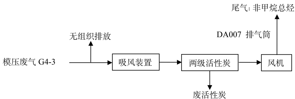
图 4-5 DA009 排气筒废气处理装置示意图
