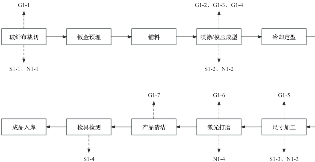
图 2-2 电池包上壳体总成、电池包下托盘底板（STM 生产线）生产工艺流程图
