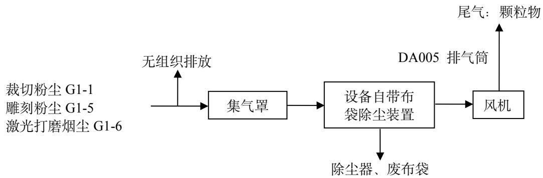
图 4-7 DA005 排气筒废气处理装置示意图
