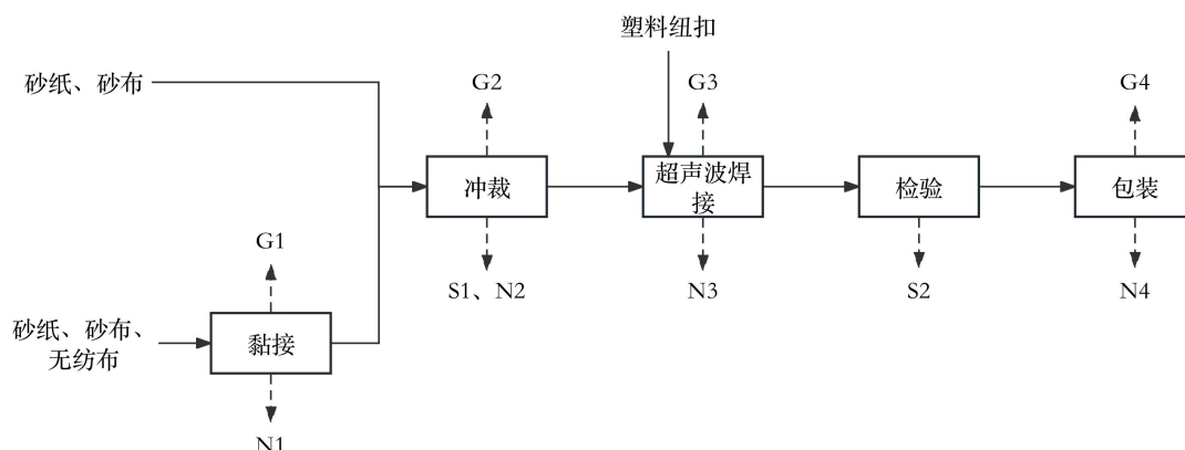
图 2-1 涂附磨具生产工艺流程图
