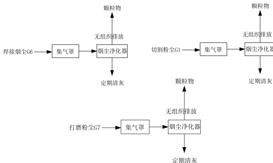
图 4.2 烟粉尘处理工艺流程图
