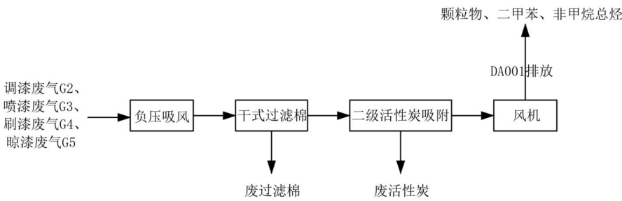
图 4.2 漆雾+有机废气处理工艺流程图
