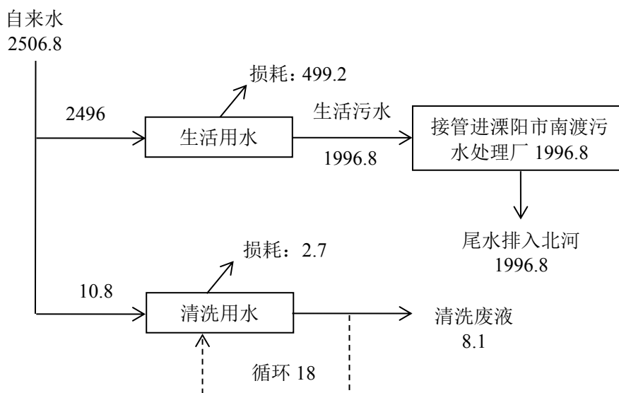
全厂水平衡图 单位：t/a
