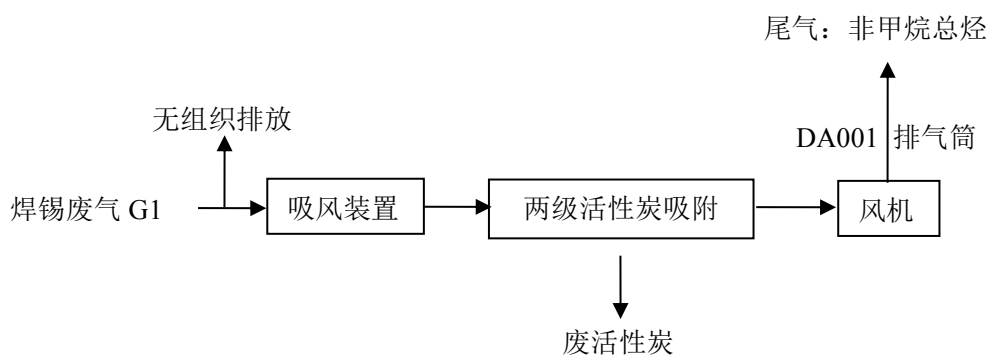
图 4-2 焊锡废气处理装置示意图
