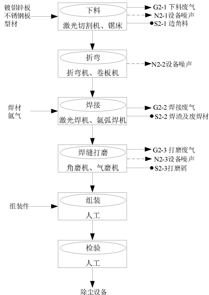
图 2-3 除尘设备生产工艺流程及产污节点图
