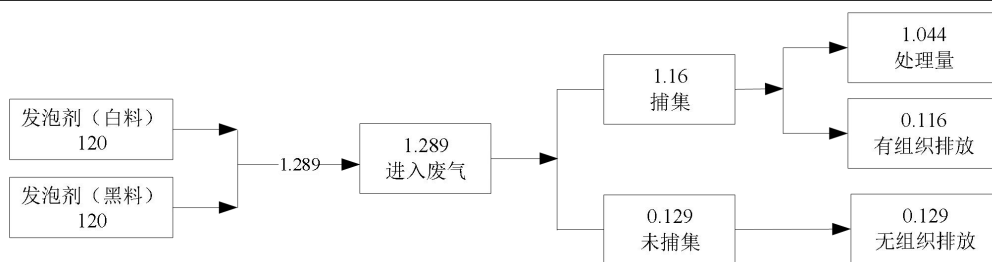
图 2-1 项目 VOCs 平衡图 (t/a)
