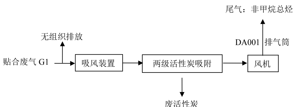
图 4-2 贴合废气处理装置示意图
