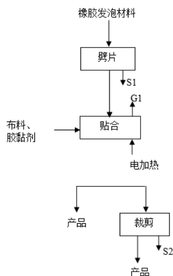
图 2-2 企业原有项目生产工艺流程图
