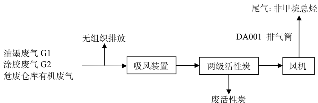
图 4-2 DA001 排气筒废气处理装置示意图
