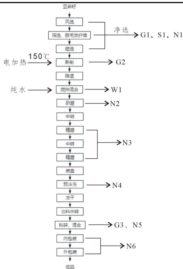
图 2-2 纯亚麻籽微粉生产工艺流程图
