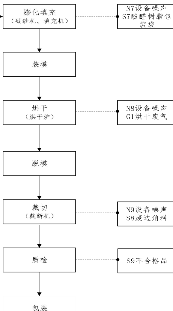
图 2-8 成型管件生产工艺流程图
