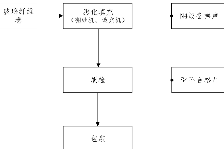
图 2-6 填充棉生产工艺流程图
