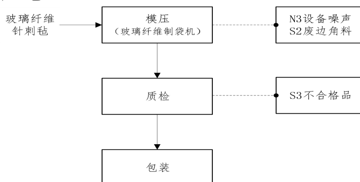
图 2-5 隔热棉生产工艺流程图
