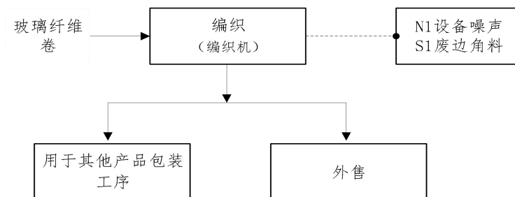
图 2-3 编织袋生产工艺流程图
