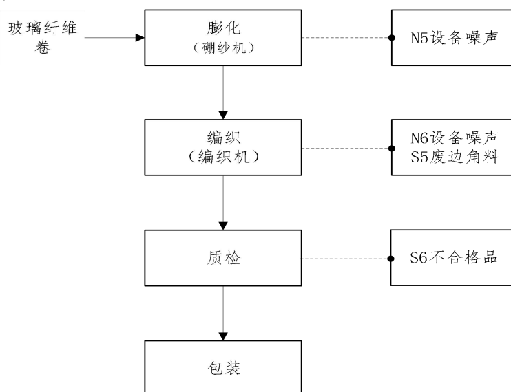
图 2-7 编织棉生产工艺流程图
