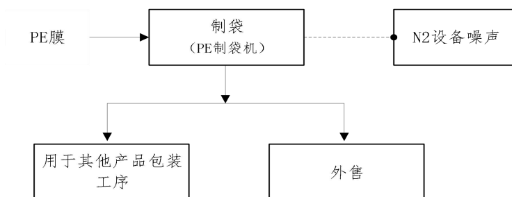
图 2-4 PE 袋生产工艺流程图
