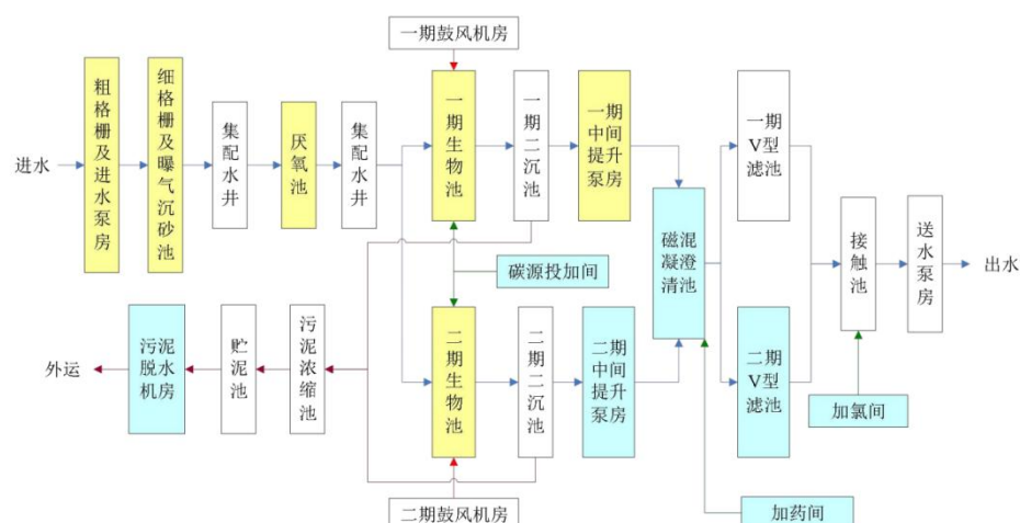
图 4-2 溧阳市第二污水处理厂处理工艺流程图
