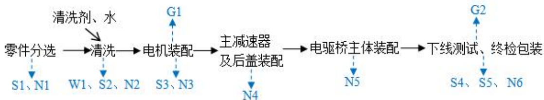
图 2-2 电驱桥组装工艺流程图
