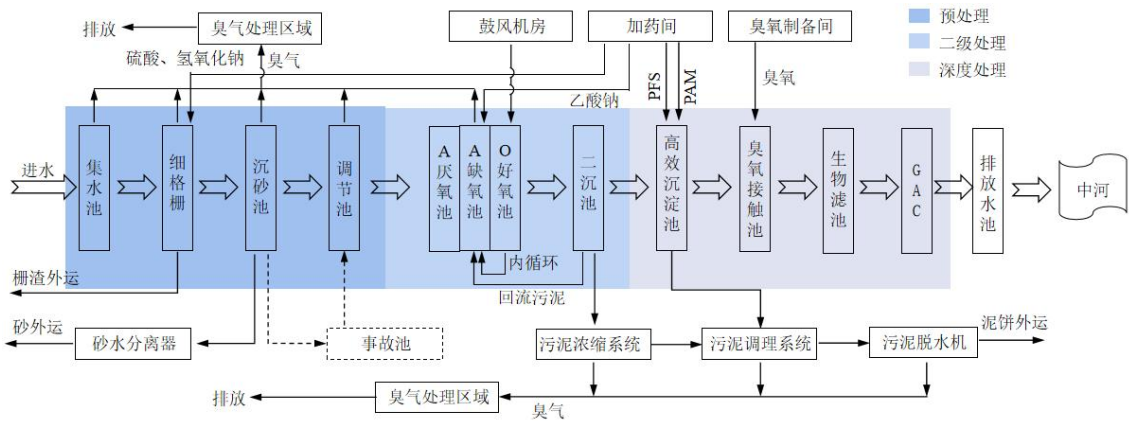
图 4-1 江苏中关村工业污水处理厂污水处理工艺流程图
