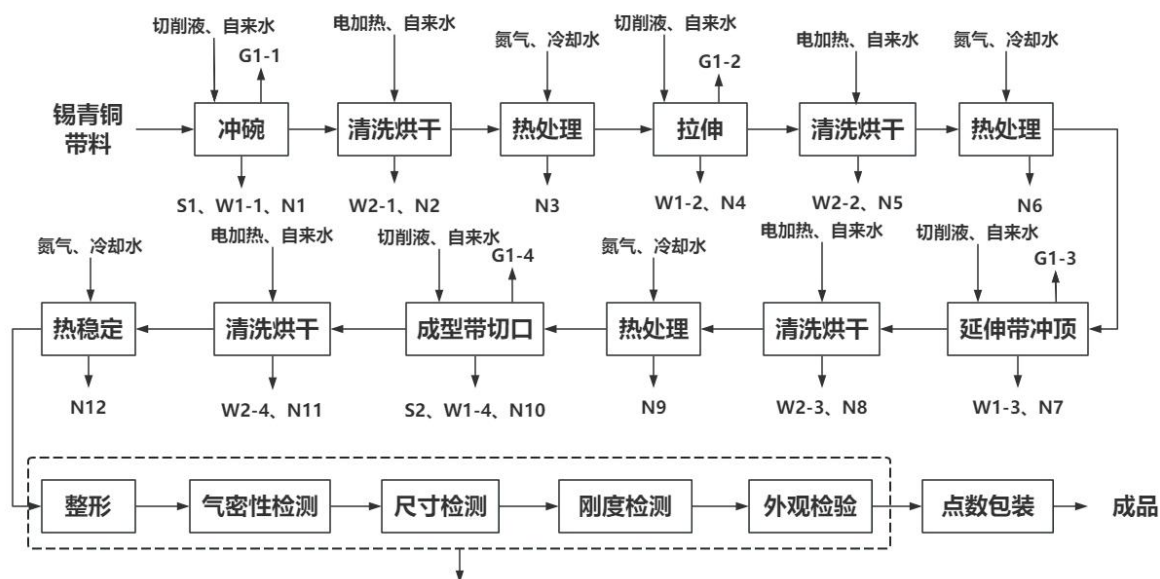
图 2-2 金属器件制作工艺流程图
