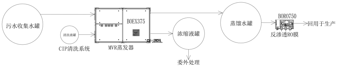
图 4-1 生产废水处理设施工艺流程图
