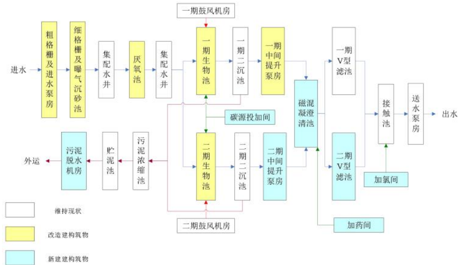
图 4-2 溧阳市第二污水处理厂处理工艺流程图
