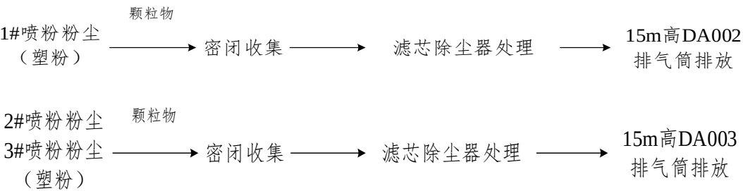
图 4-2 喷粉粉尘（塑粉）废气处理流程图
