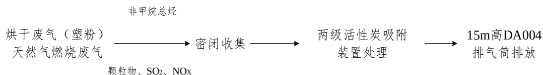
图 4-3 烘干废气（塑粉）、天然气燃烧废气处理流程图
