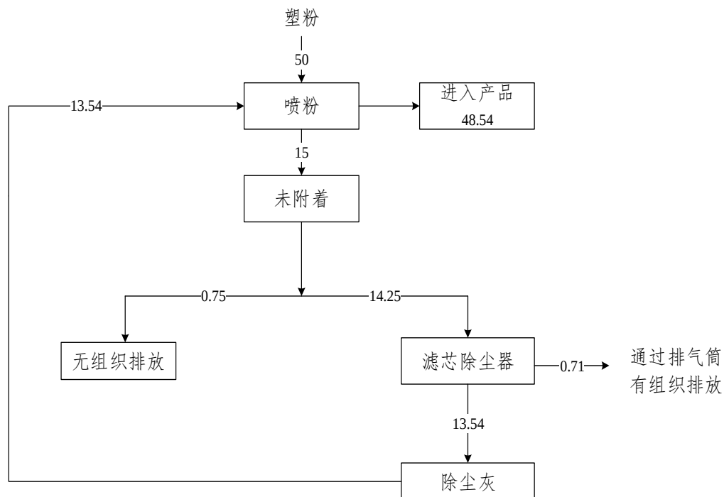
图 2-2 项目塑粉平衡图 t/a
