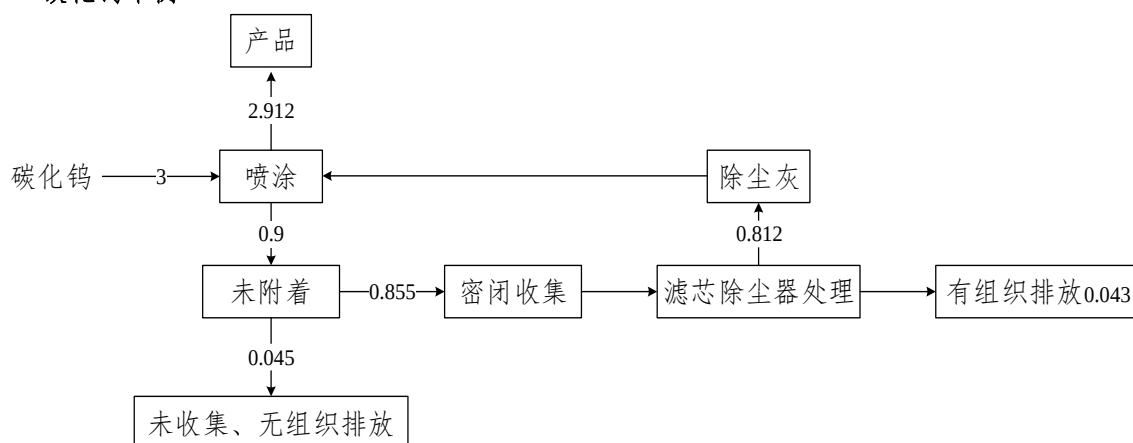
图 2-3 项目碳化钨平衡图 t/a
