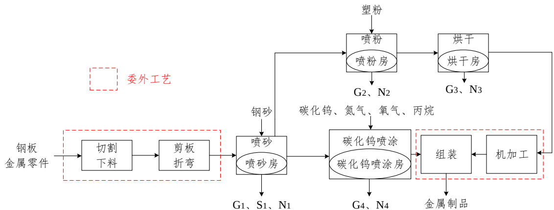
图 2-2 金属制品生产工艺流程及产污节点图
