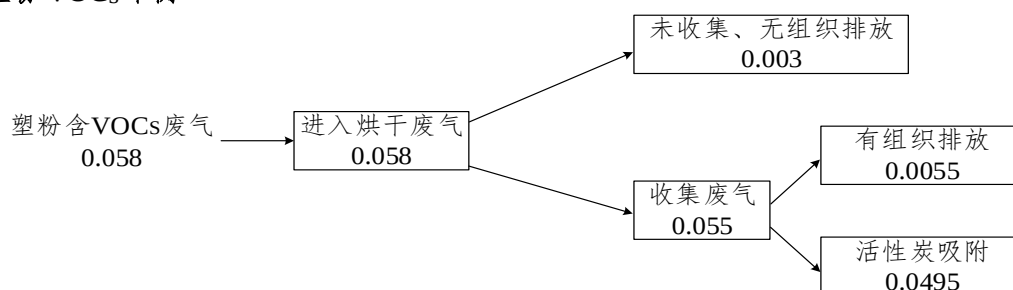
图 2-4 塑粉 VOCs 平衡图 t/a
