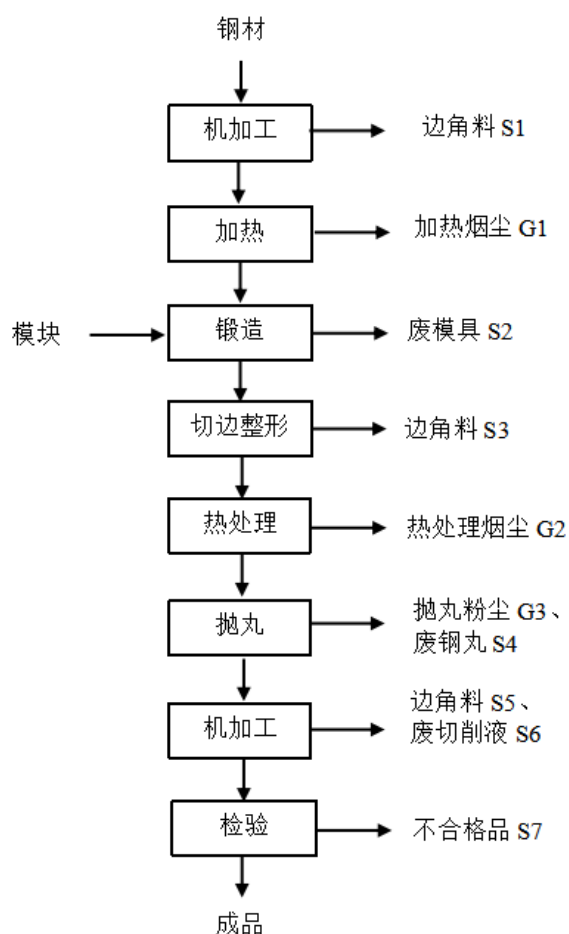
图 2-4 生产工艺流程图
