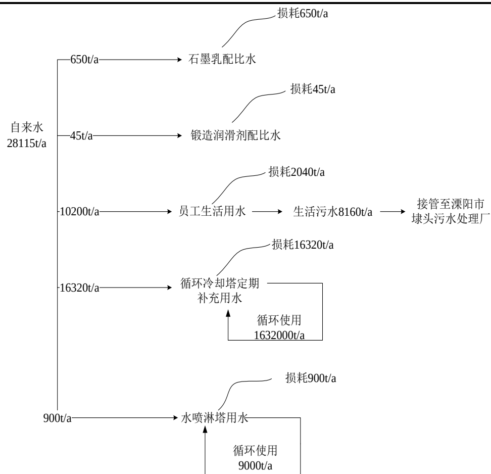
图 2-2 技改后全厂水平衡图
