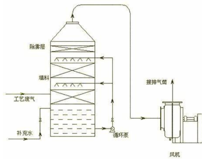
图 4-2 水喷淋塔结构示意图
