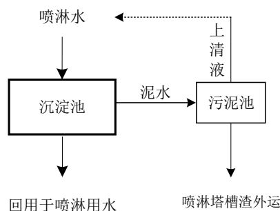
图 4-1 喷淋水处理工艺流程图
