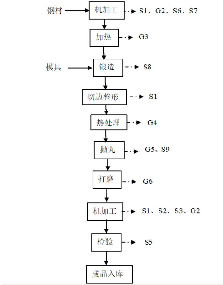
图 2-5 汽车零部件生产流程图
