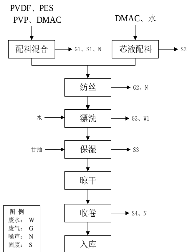
图 2-2 塑料丝生产工艺流程图及产污节点图
