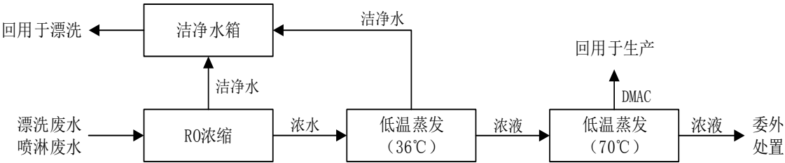
图 4-5 回用水处理设施工艺流程图
