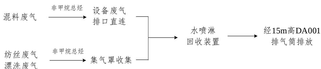
图 4-3 有机废气处理工艺流程图
