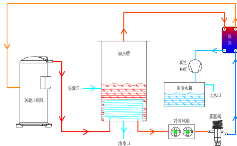
图4-4 低温蒸发流程图
