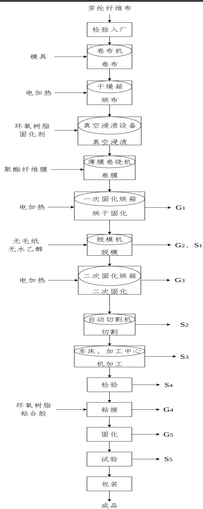
图 2-3 原有项目生产工艺流程及产污节点图
