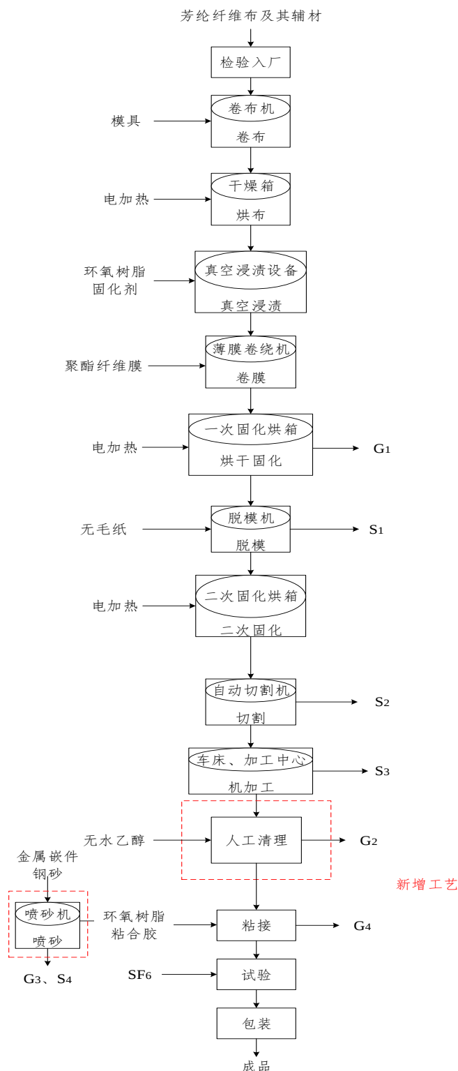
图 2-2 高压绝缘拉杆生产工艺流程及产污节点图
