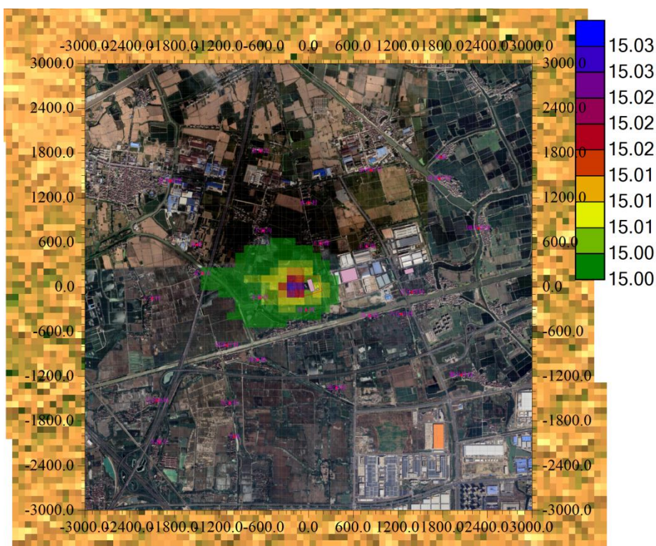
图 5.2.1.6-6 SO 2 叠加现状浓度后最大 98%保证率日均浓度分布图
