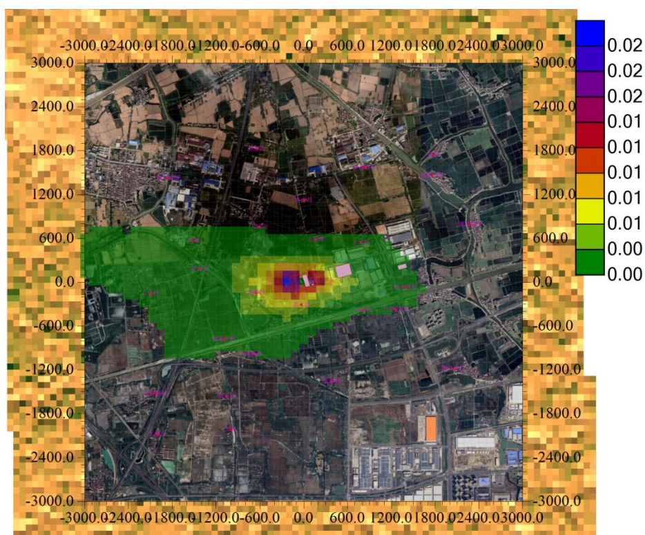
图 5.2.1.6-7 SO 2 最大年均浓度贡献值分布图
