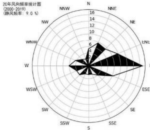
图 4.1.3-1 溧阳地区风向玫瑰图（静风频率 9.0%）
