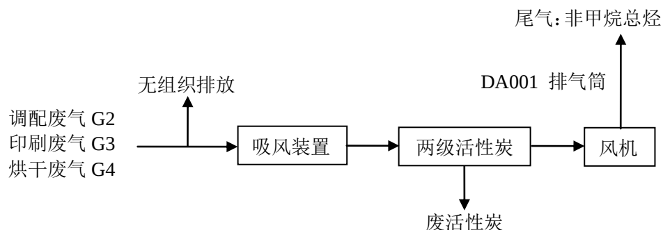
图 4-2 DA001 排气筒废气处理装置示意图
