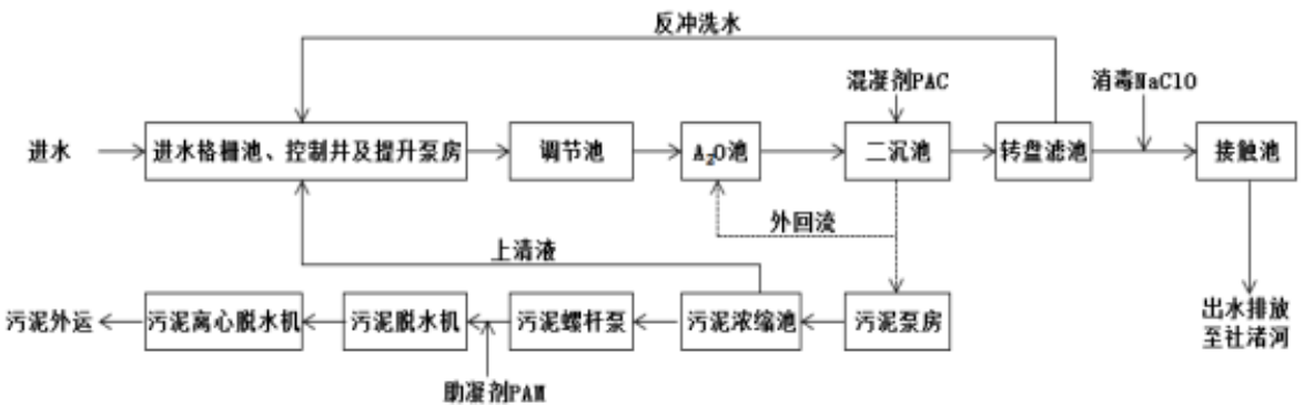
图 4-1 溧阳市社渚污水处理厂处理工艺流程图
