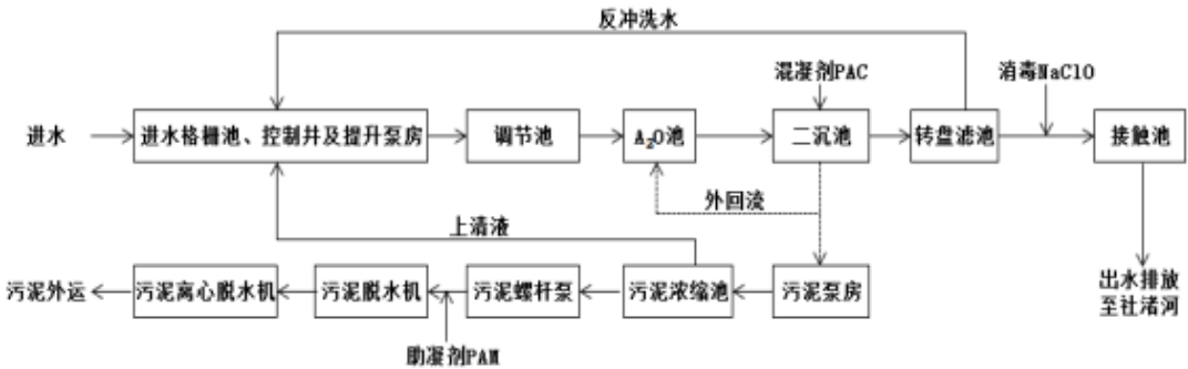
图 1-1 污水处理工艺流程图
