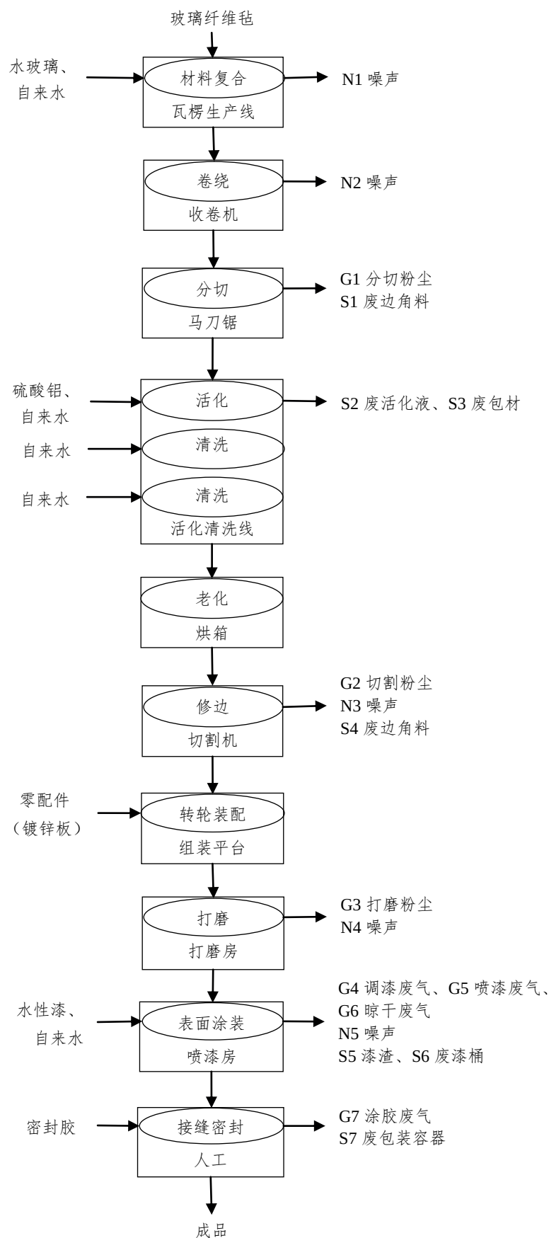
图 2-2 除湿转轮生产工艺流程图
