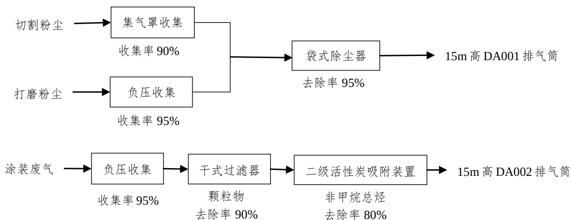
图 4.1-1 切割粉尘、打磨粉尘收集处理流程图
