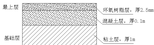
图 4.5-1 重点防渗区域剖面图
